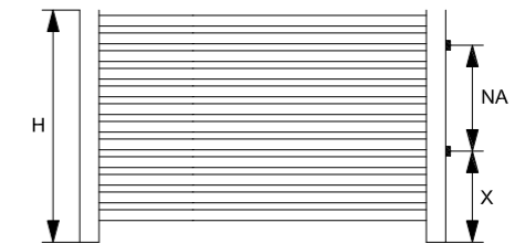
Seitenanschluss rechts
